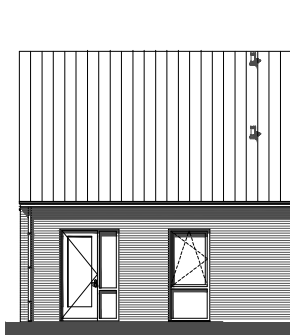
Achtergevel 1:200
