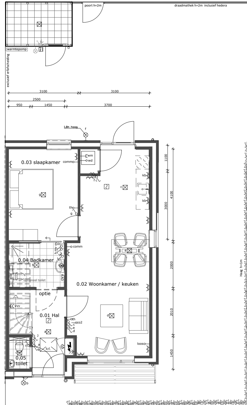
Begane grond 1:100
