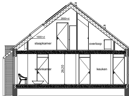
Doorsnede 1:200
