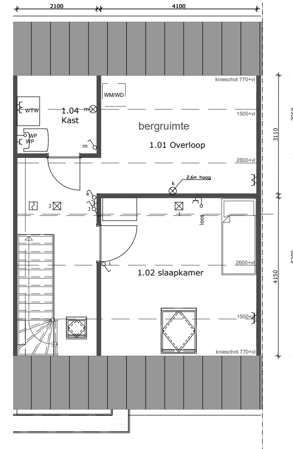
1e verdieping 1:100
