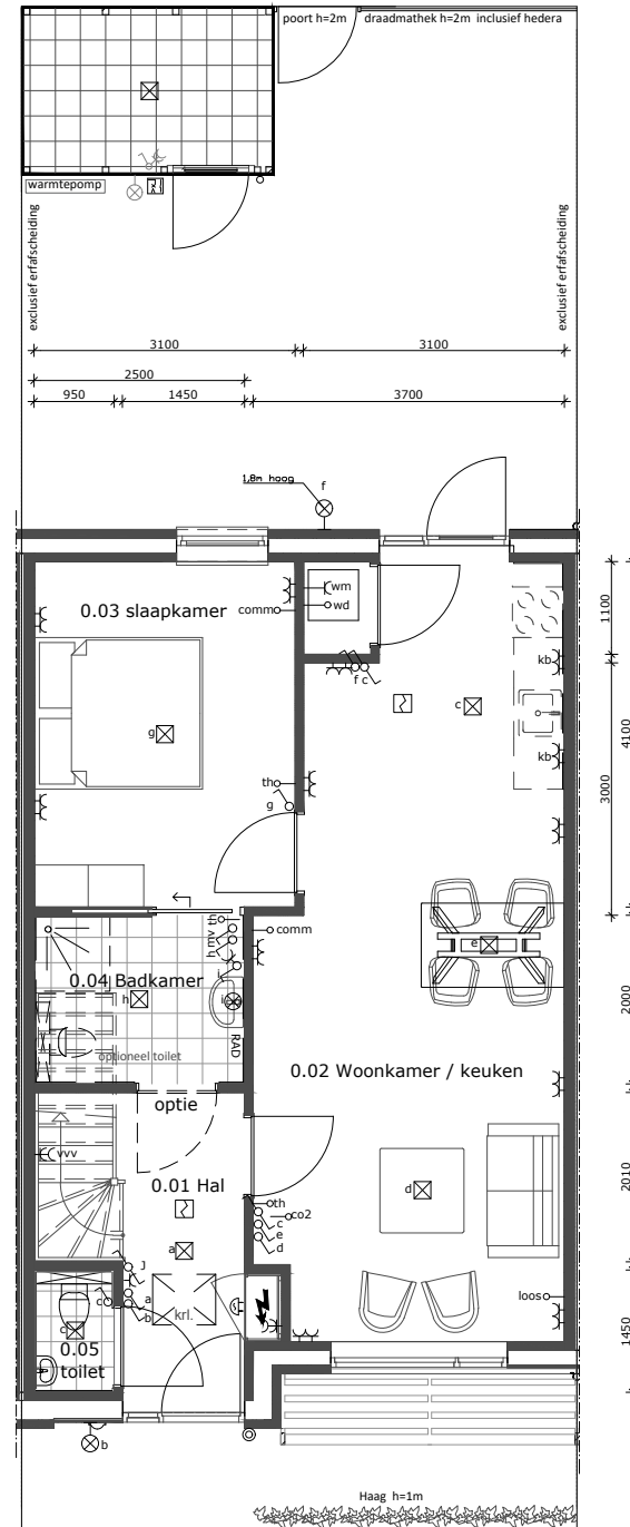
Begane grond 1:100
