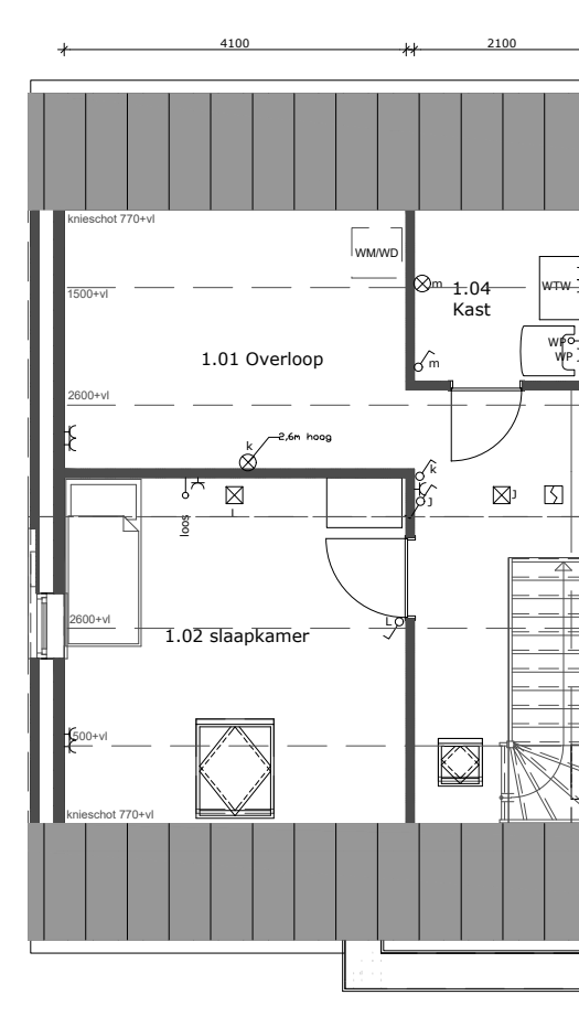
1e verdieping 1:100
