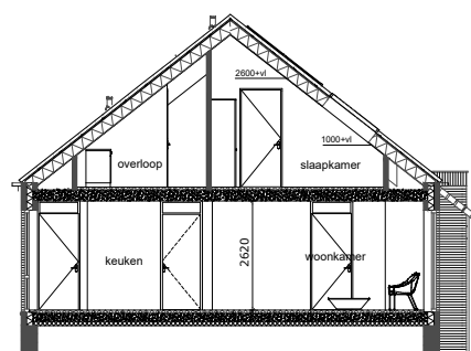
Doorsnede 1:200
