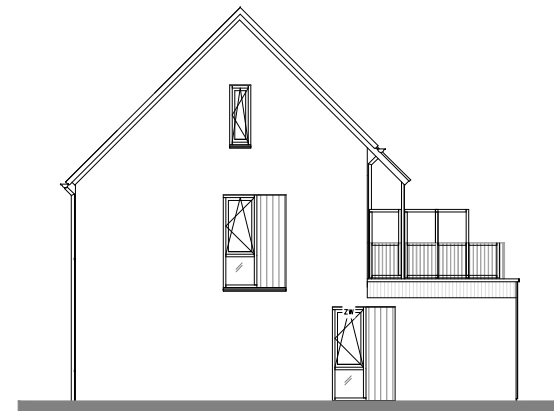
Linker zijgevel 1:200
