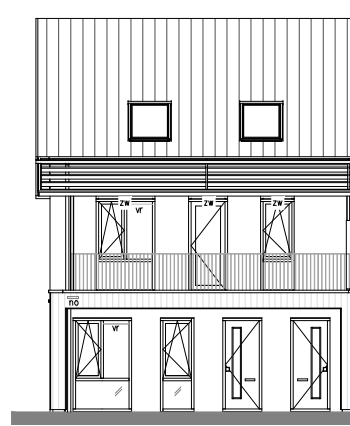
Voorgevel 1:200
