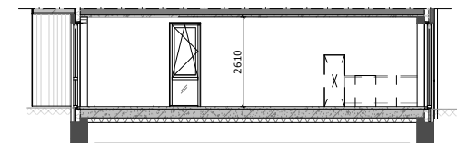
Doorsnede 1:200
