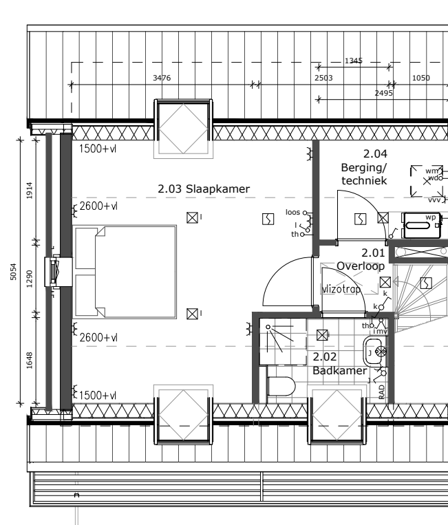
2e verdieping 1:100
