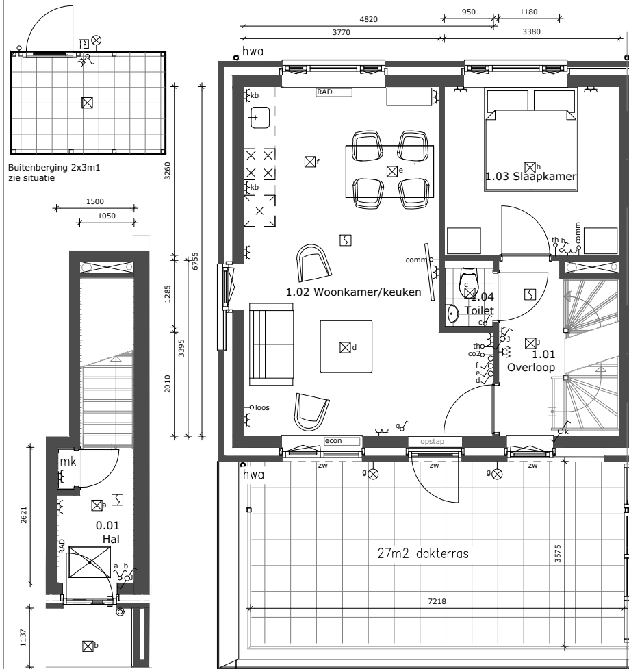
begane grond 1:100
