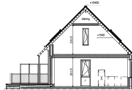
Doorsnede 1:200
