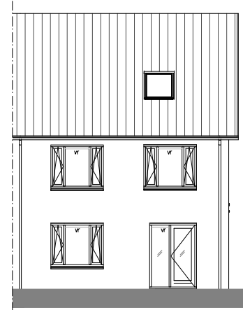
Achtergevel 1:200
