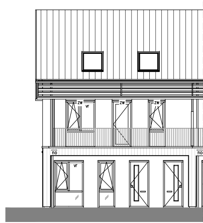
Voorgevel 1:200
