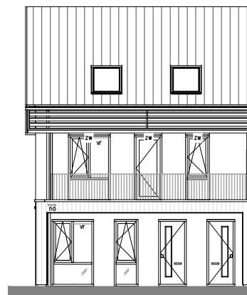
Voorgevel 1:200
