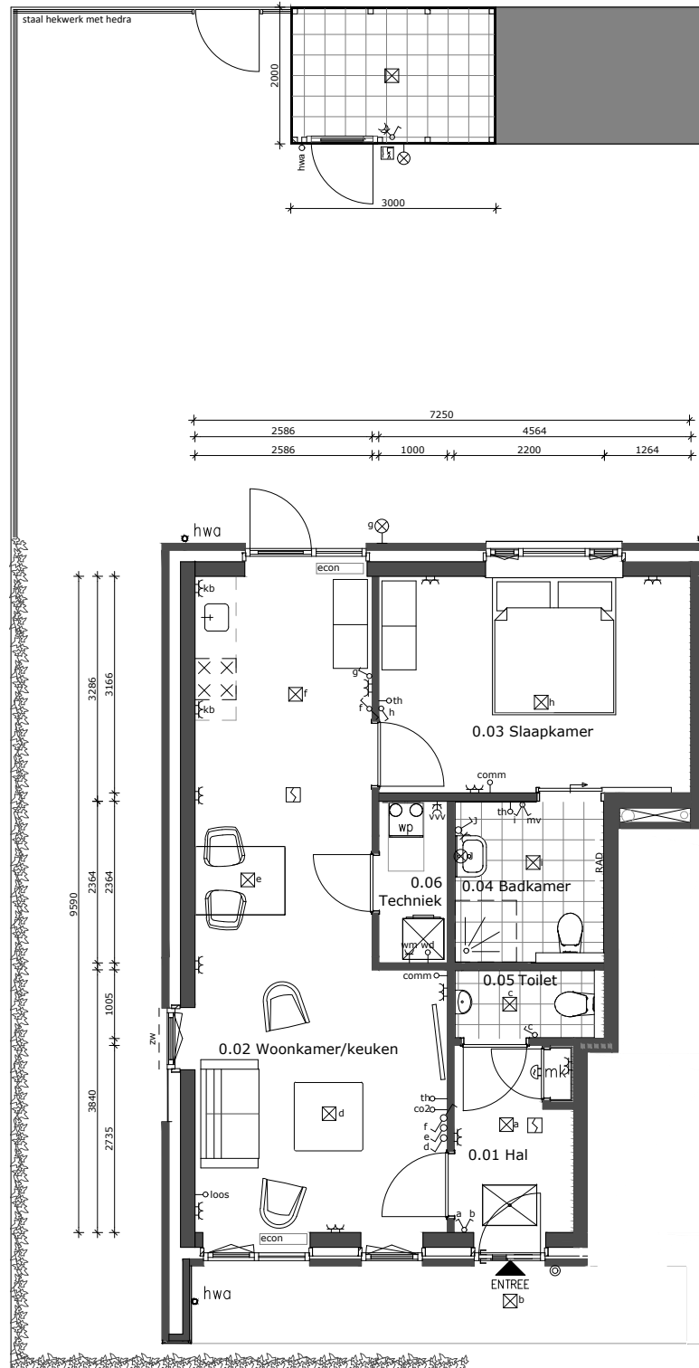
Begane grond 1:100
