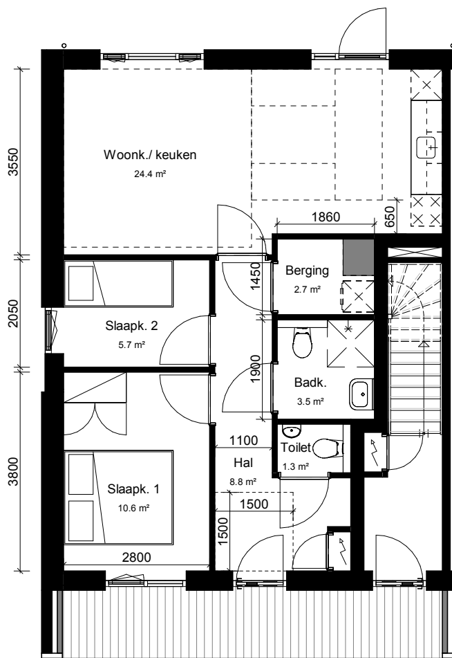
begane grond 1:100
